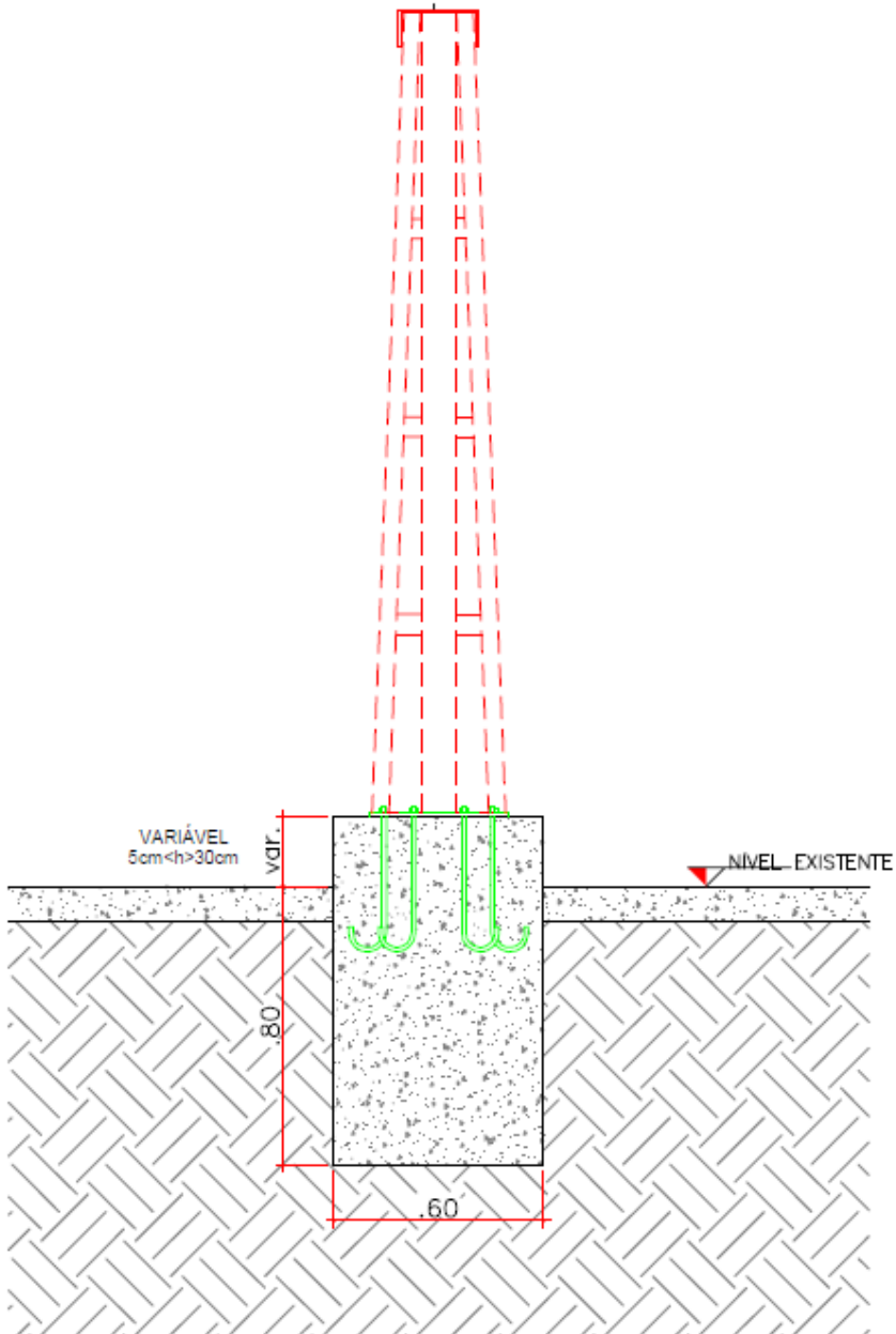
ELEVAÇÃO ESCALA: 1:25
